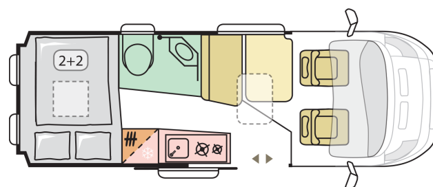
LAY-OUT NACHT
