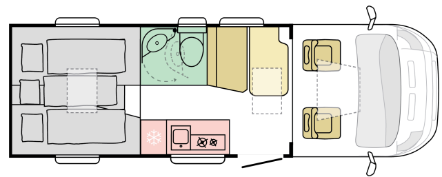
LAY-OUT NACHT
